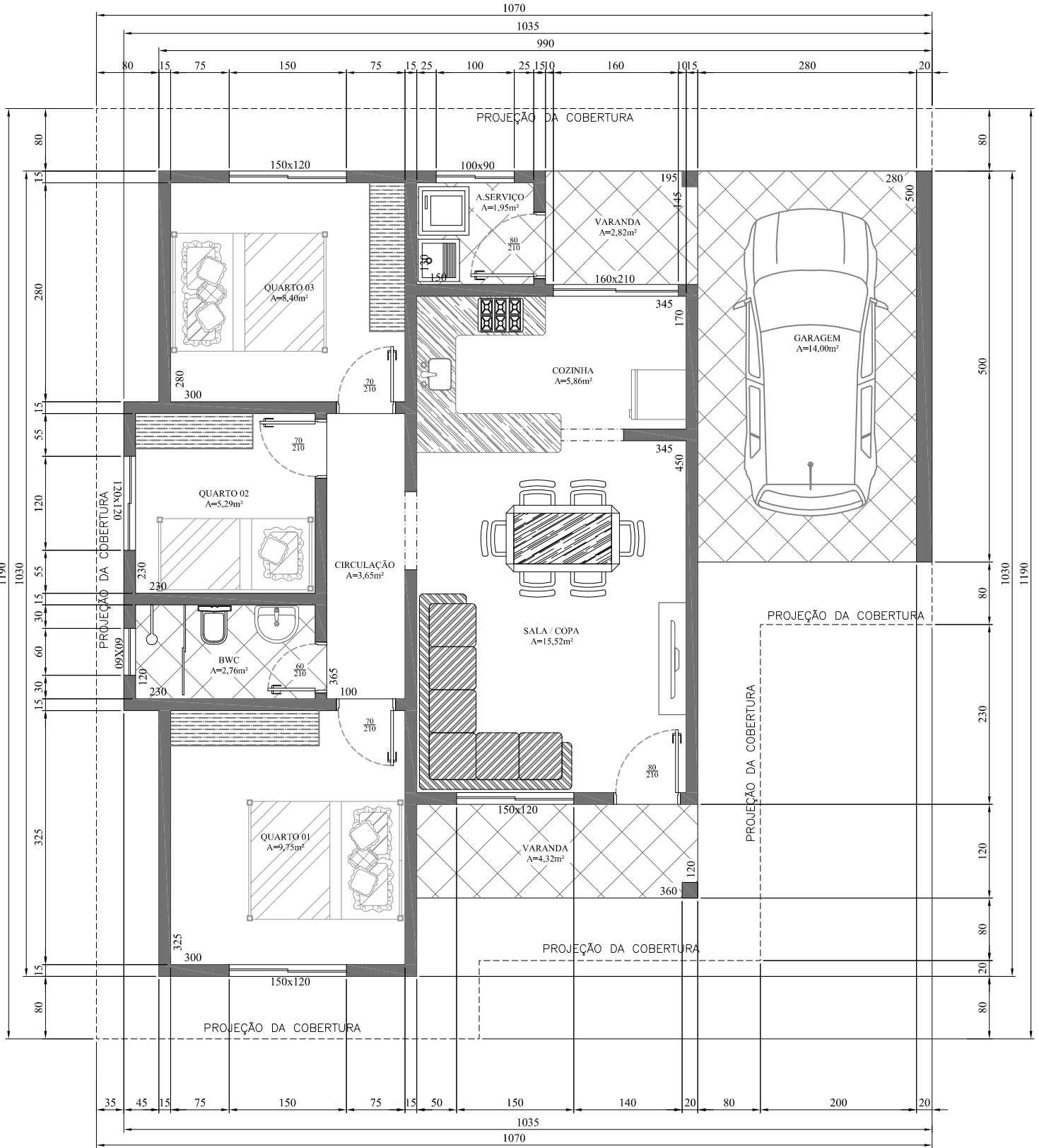
PLANTA BAIXA A= 85,00m 2
